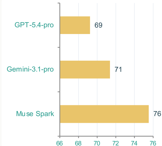
MultiChallenge
