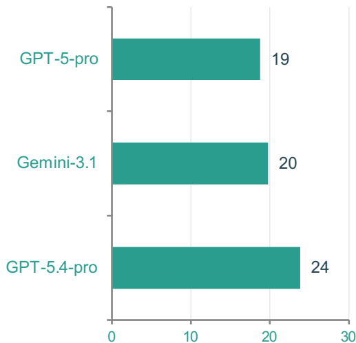
EnigmaEval
