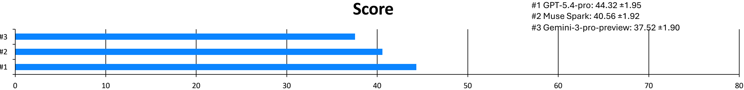
HLE — Top 3
