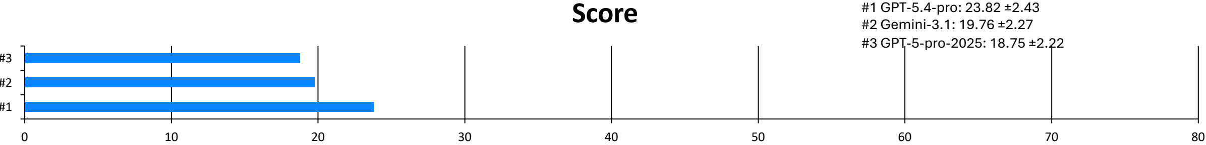
EnigmaEval — Top 3
