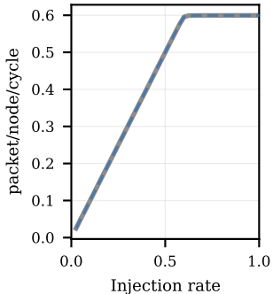
Y-Tornado: reception
