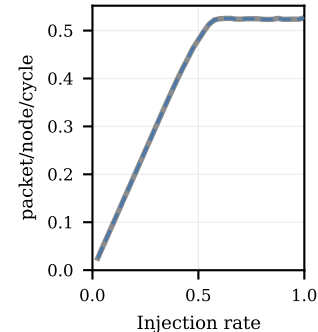
X-Tornado: reception
