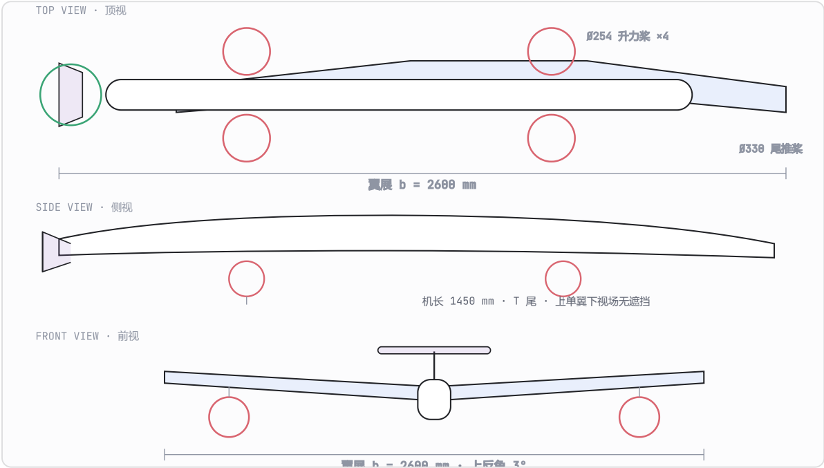
图 2-1 翎雁 LY-100 三视图（顶视 / 侧视 / 前视 · 示意，公差与详图见配套图纸包）
