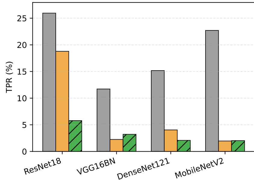
LiRA TPR@1%FPR
