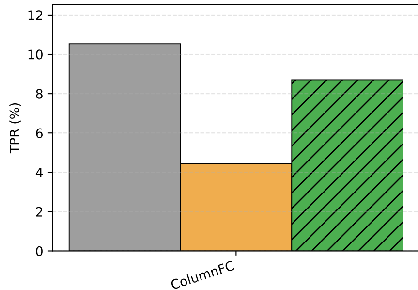
LiRA TPR@1%FPR
