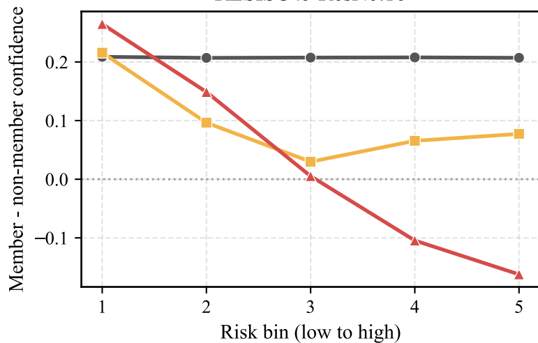
RESISC45 ResNet18
