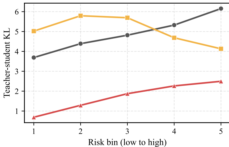
RESISC45 ResNet18
