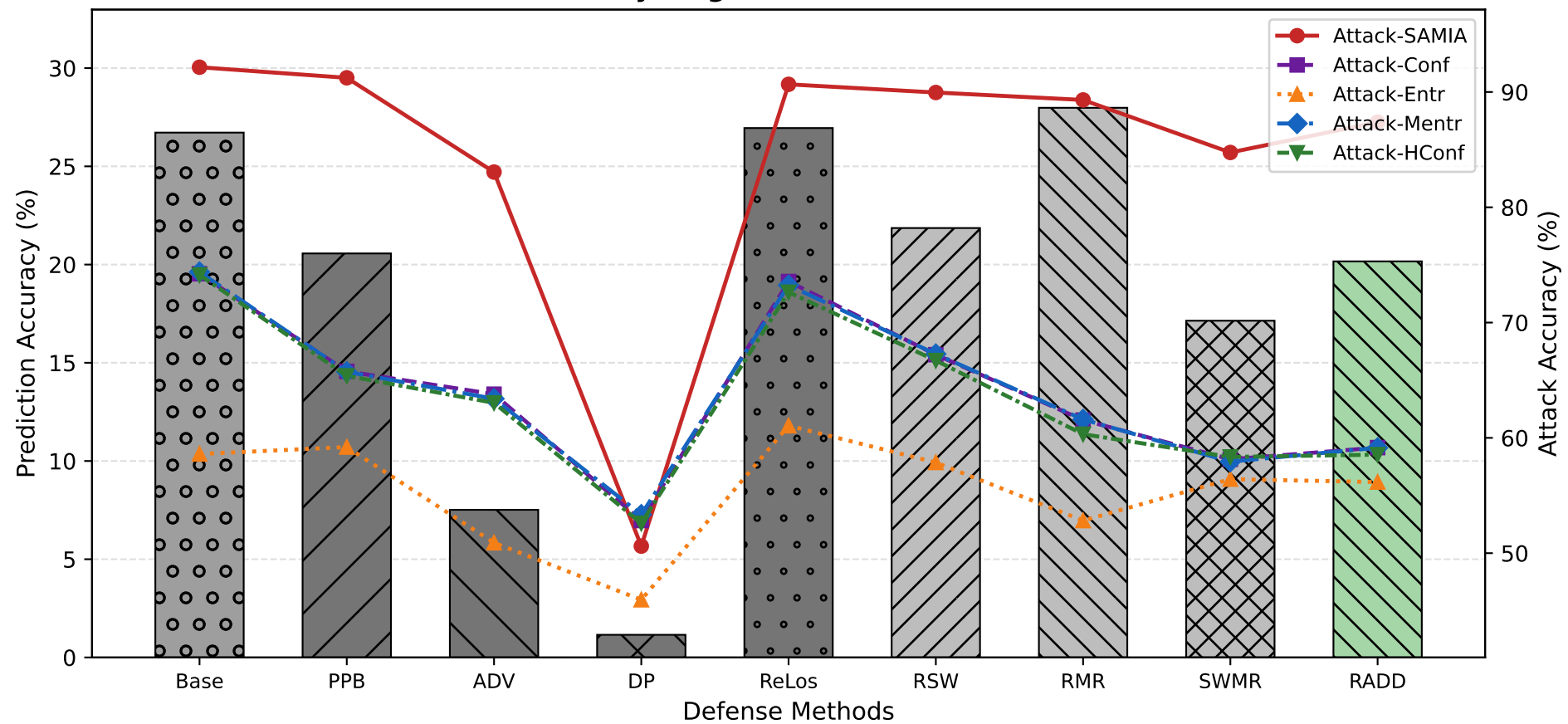
(Tinyimagenet Mobilenetv2)
