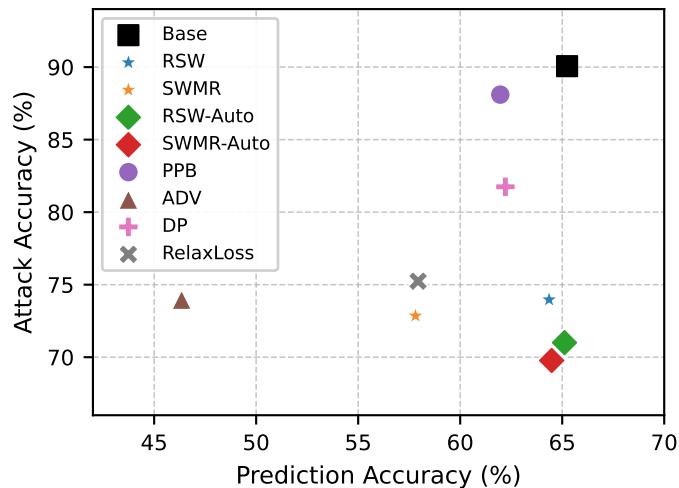
(d) FC (SAMIA)
