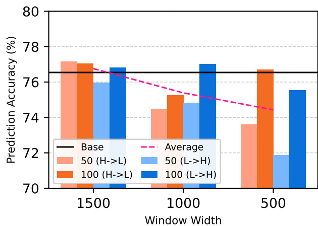
(b) CIFAR10 Res18 (SWMR)
