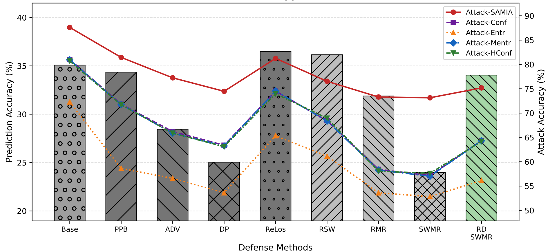
(Cifar100 Vgg16bn)
