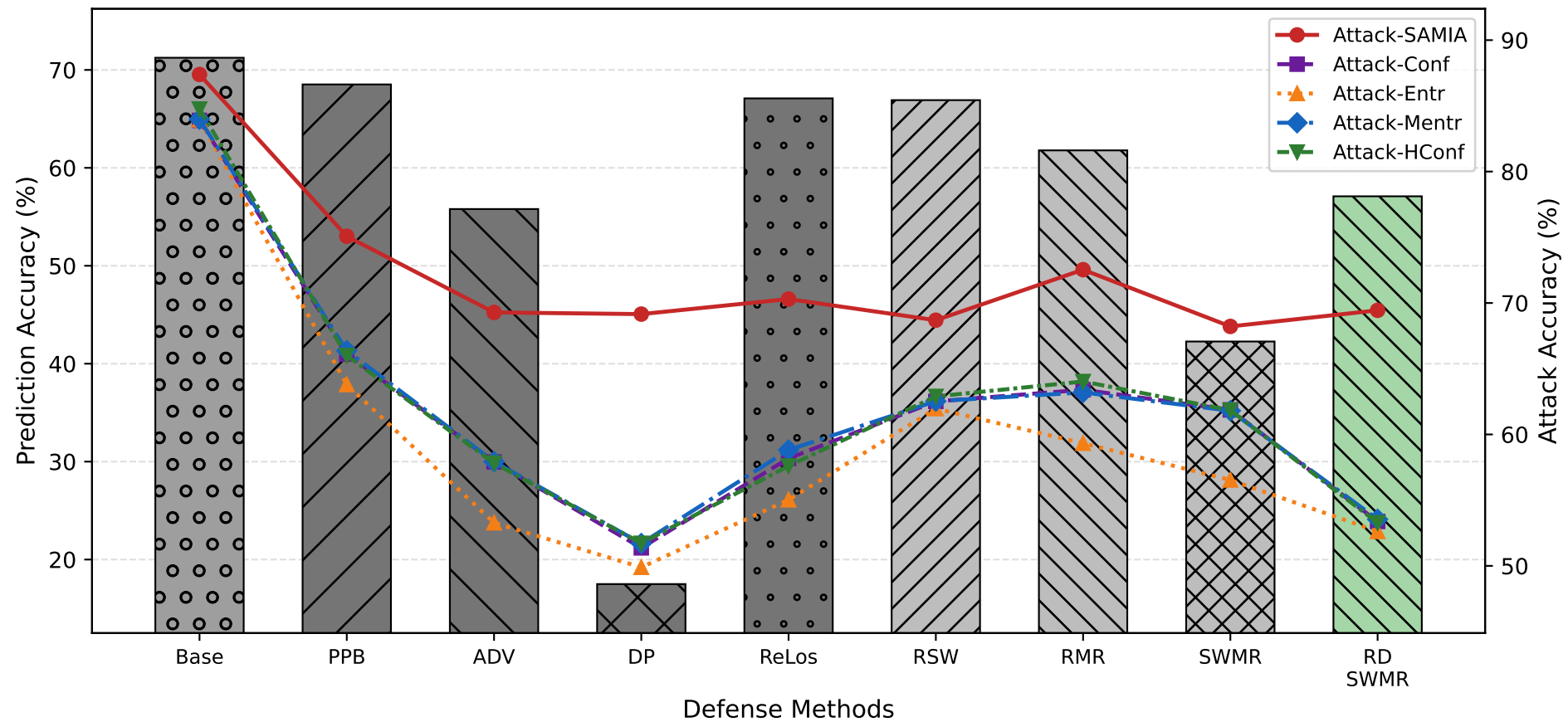
(Resisc45 Resnet18)
