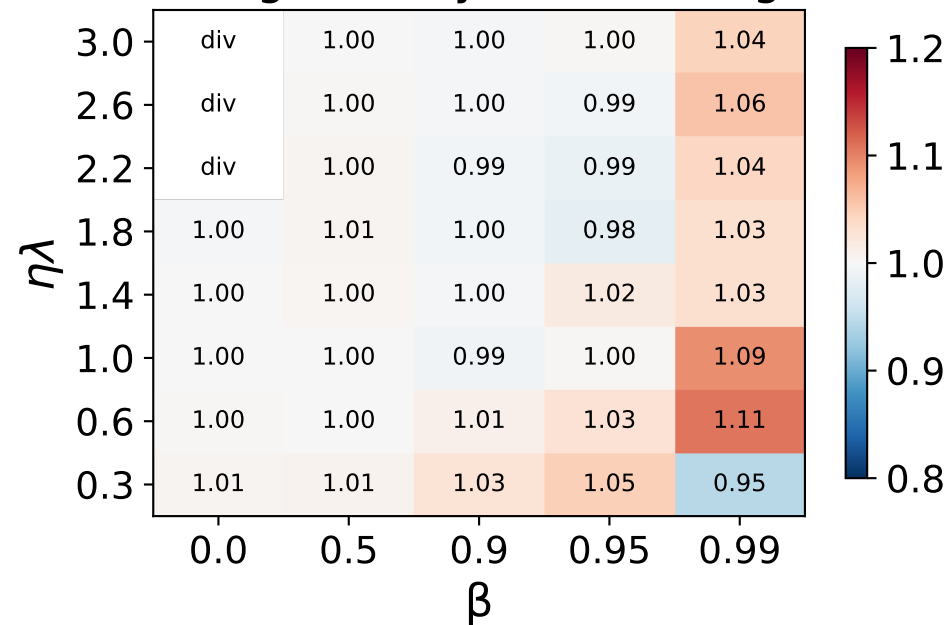
(a) straight valley: rms / CL-2 guide
