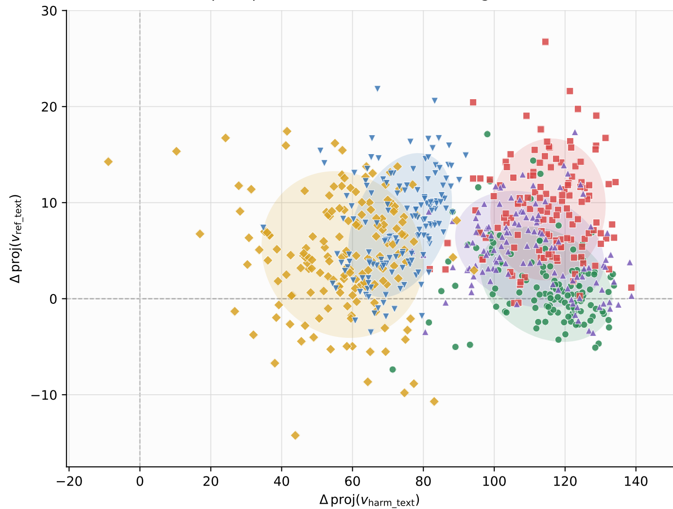
prompt-side: Qwen3-VL-4B-Thinking, L32
