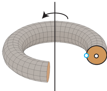
(b) Torus
