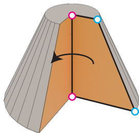
(d) Cone
