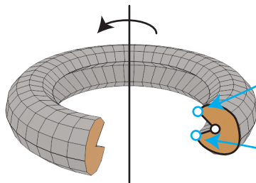
(e) Torus
