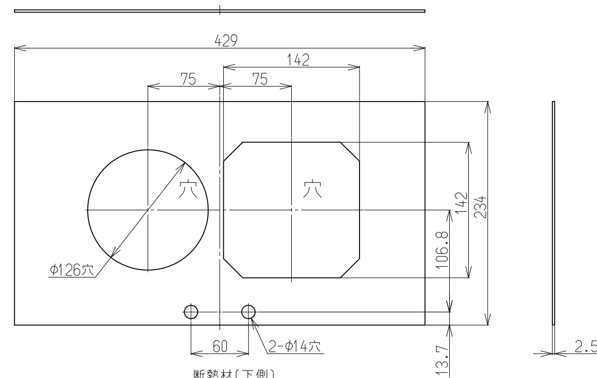
断熱材(下側)
