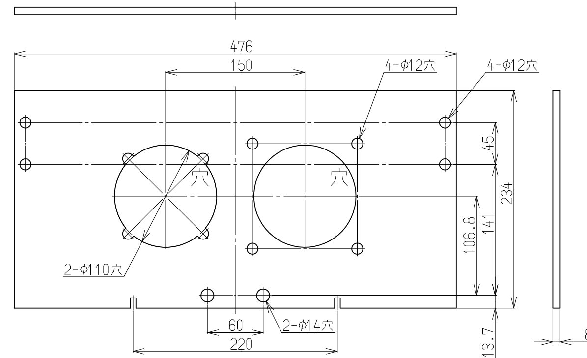
断熱材(上側)
