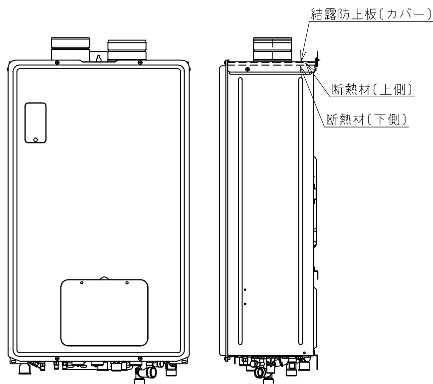
結露防止板取付図
