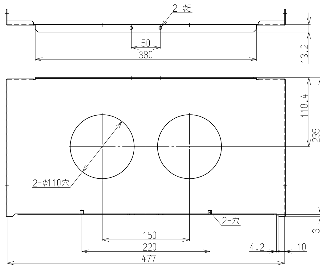
結露防止板(カバー)
