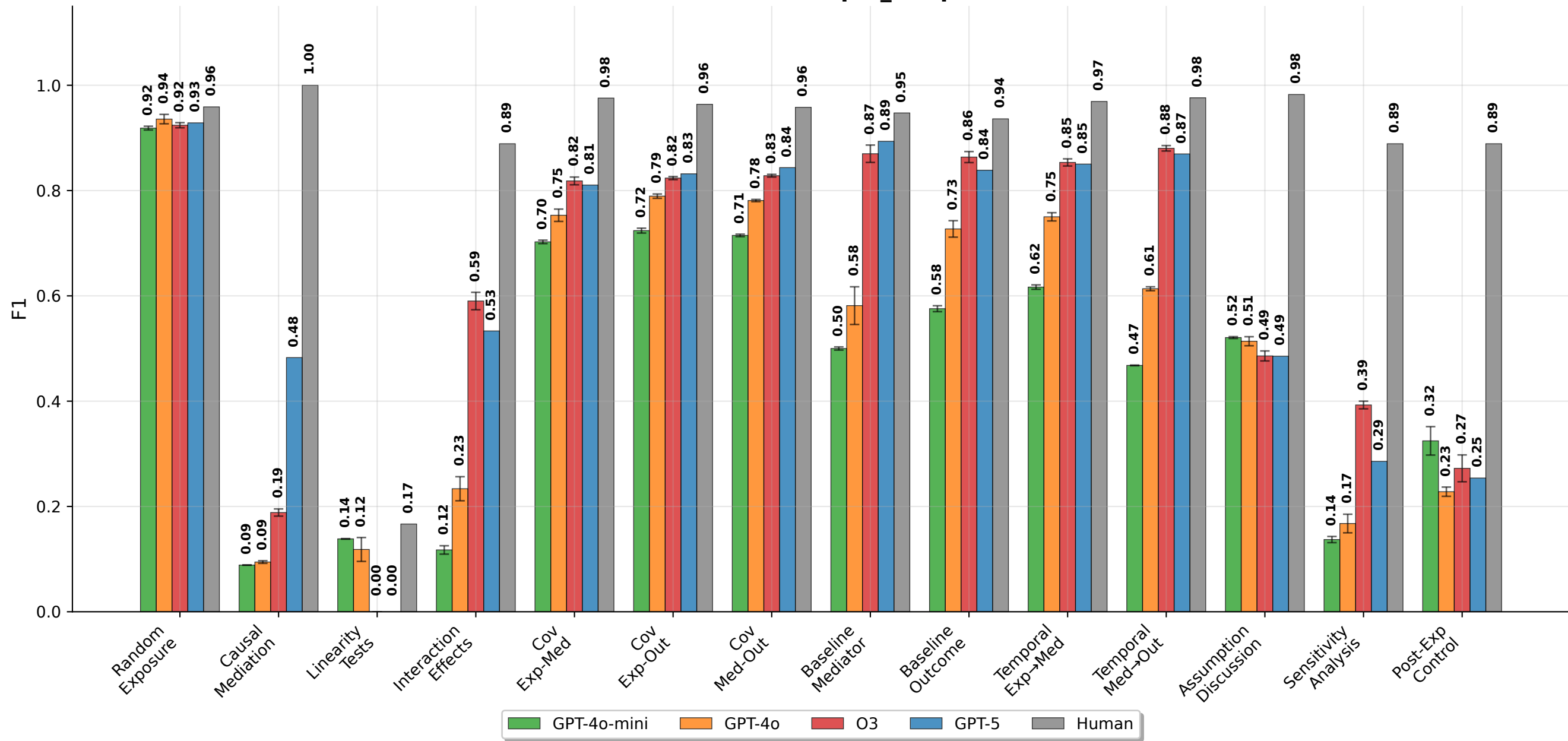
F1 - Basic Prompts_temp1.0
