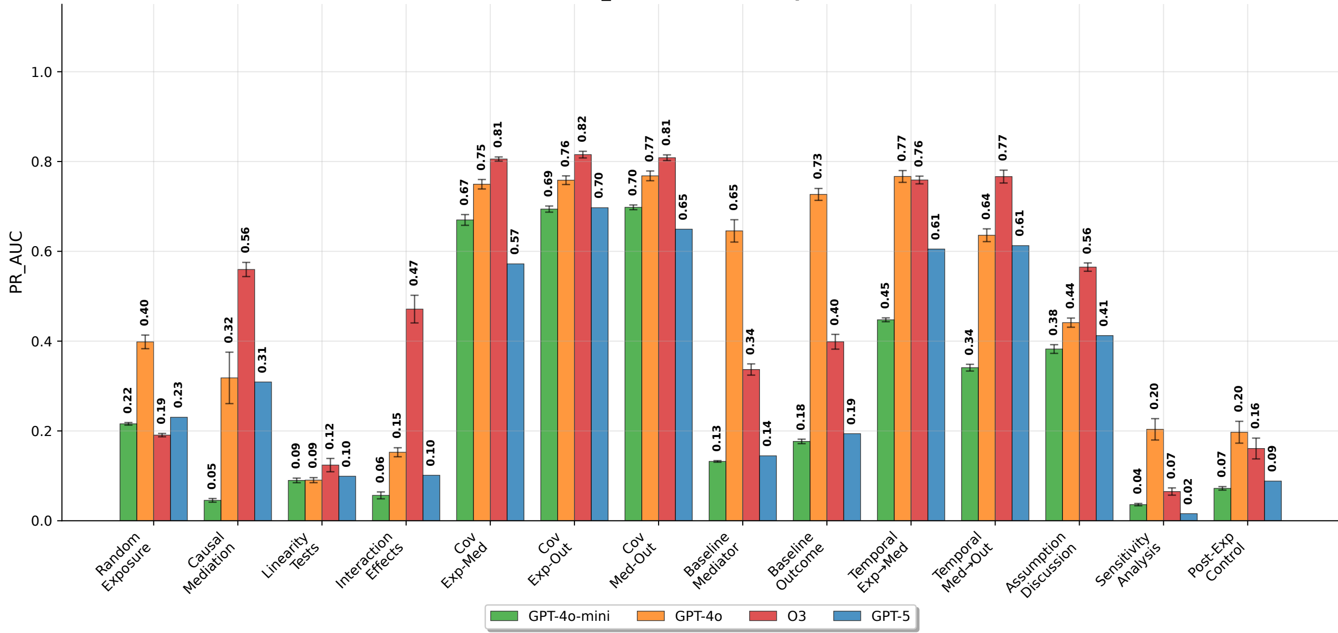
PR_AUC - Basic Prompts
