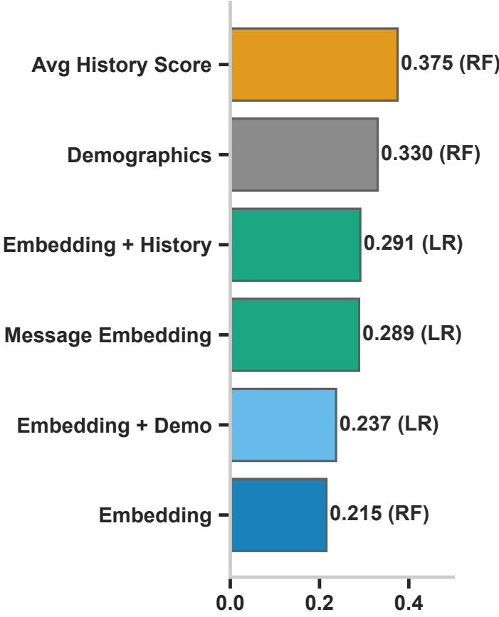
Content | F1
