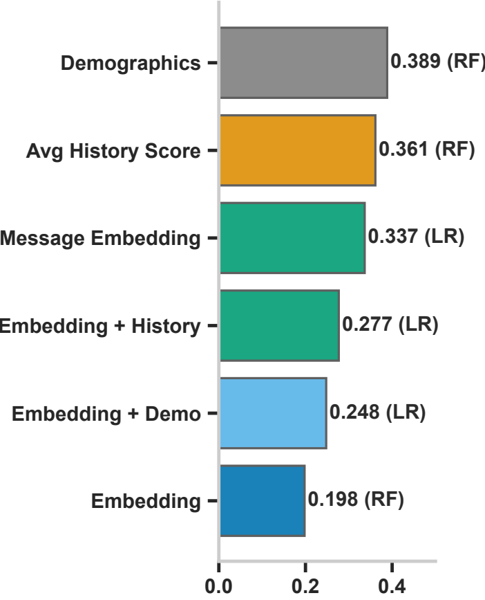
Coping | F1
