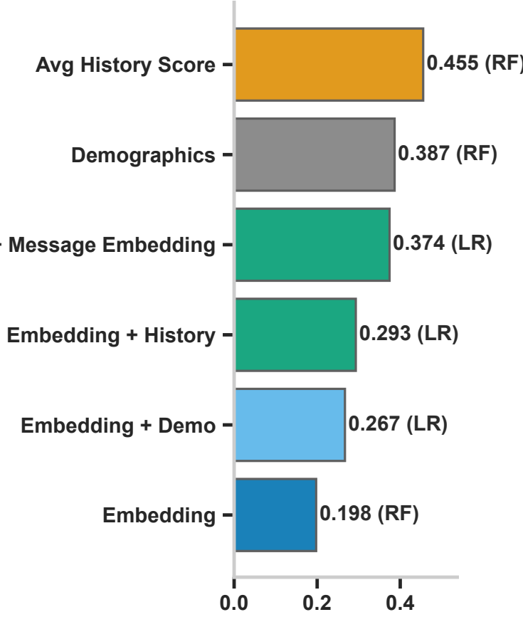
Quitting | F1
