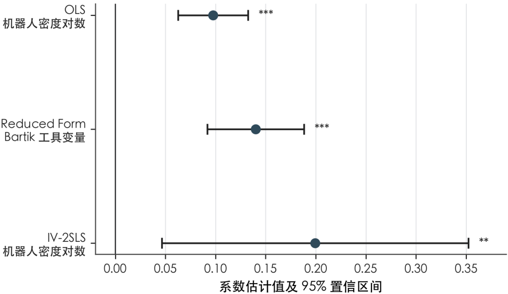
图 5-2a 工资方程：不同估计口径下的核心系数比较
