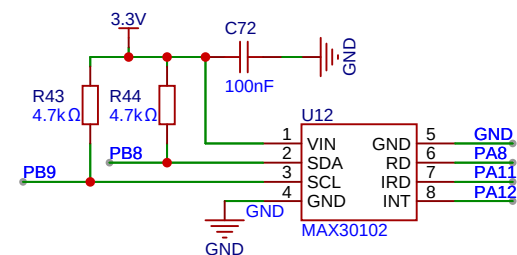
MAX30102心率传感器
