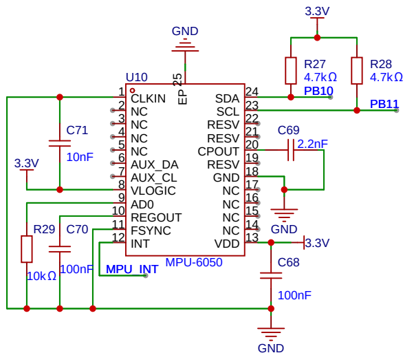
MPU6050六轴传感器
