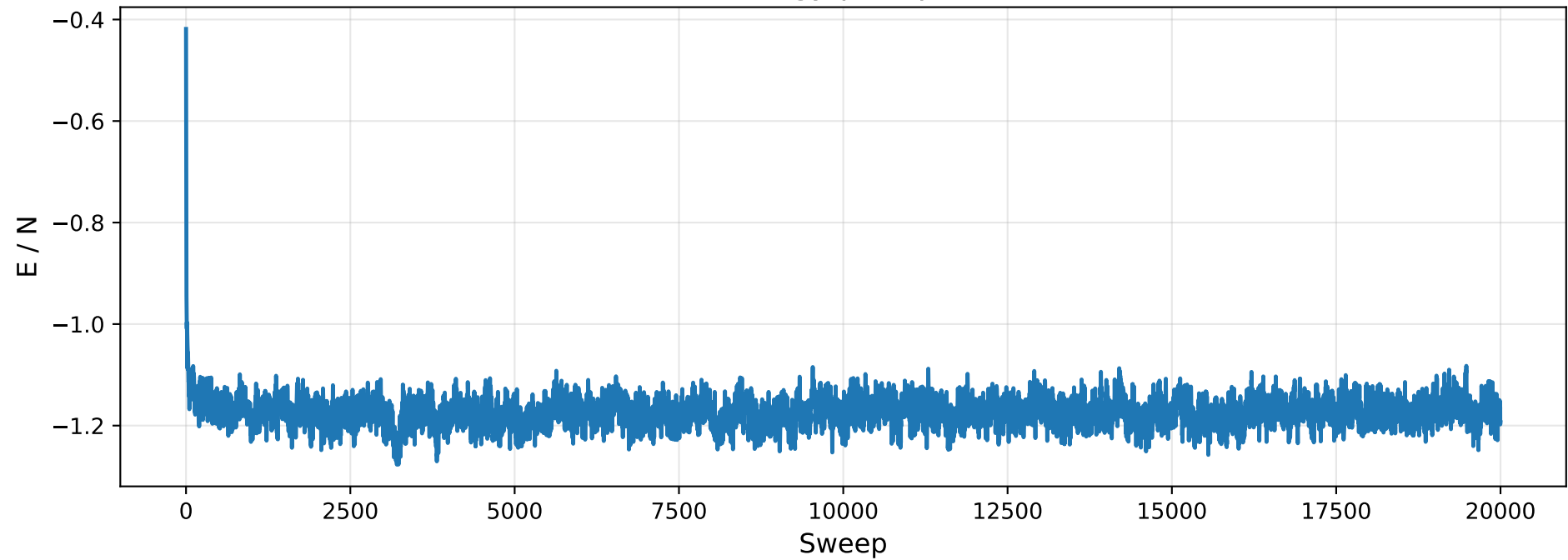
Energy per spin
