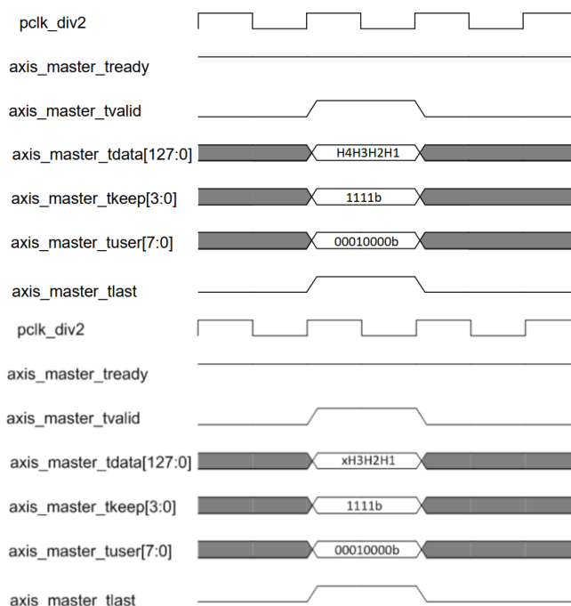
图 7 4DW/3DW Non-Posted 操作时序
