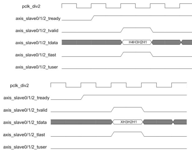
图 10 4DW/3DW Non-Posted 操作时序
