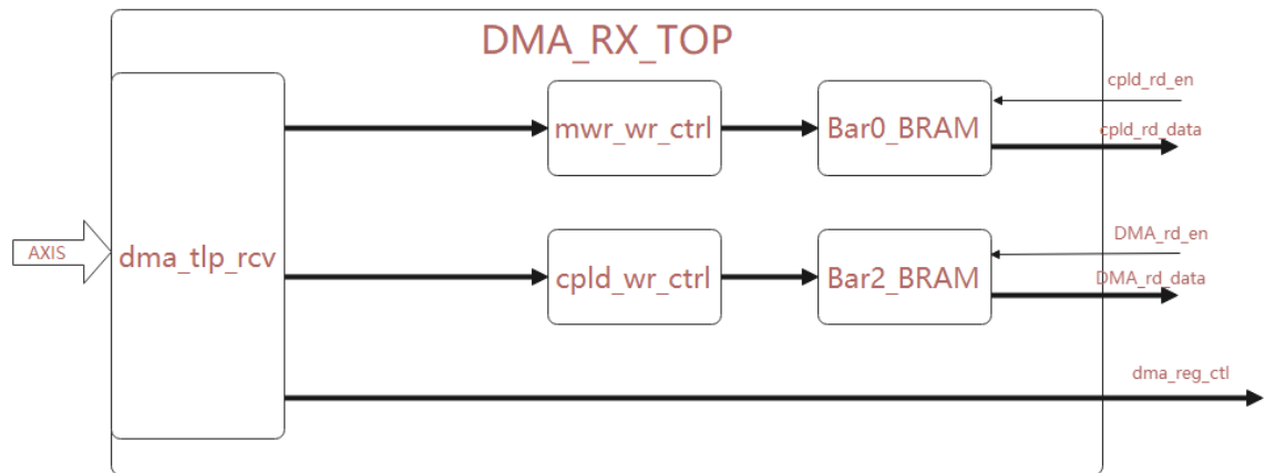
图 11 DMA_RX_TOP 模块内部框图
