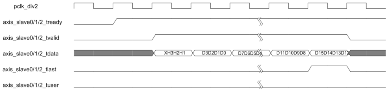
图 9 3DW Posted 操作时序
