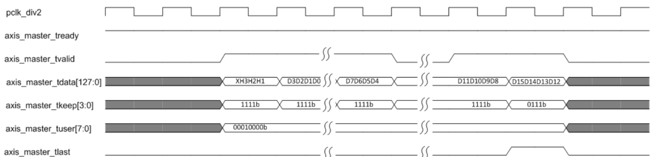
图 6 3DW Posted 操作时序
