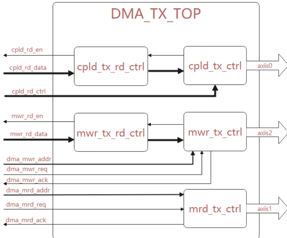
图 12 DMA_TX_TOP 模块内部框图
