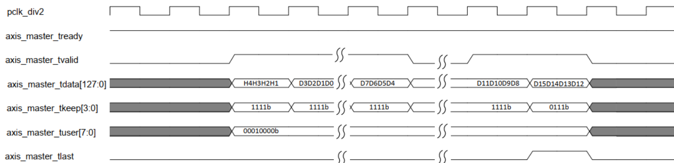
图 5 4DW Posted 操作时序
