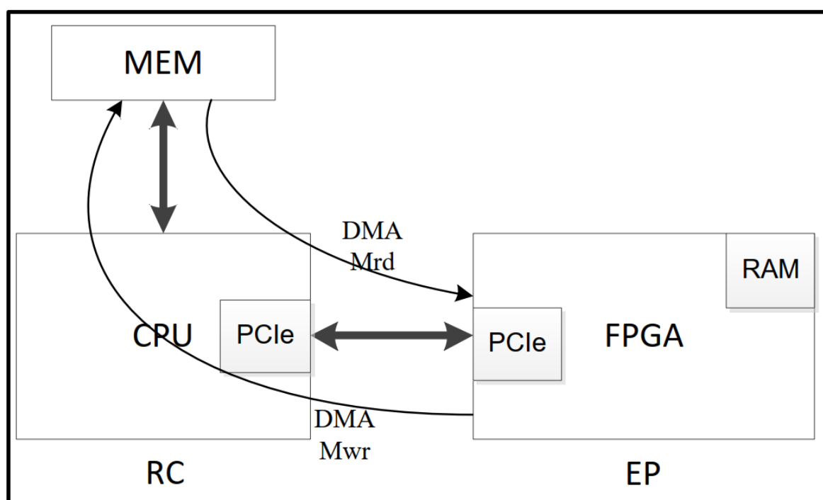
图 1 PCIe DMA 应用场景
