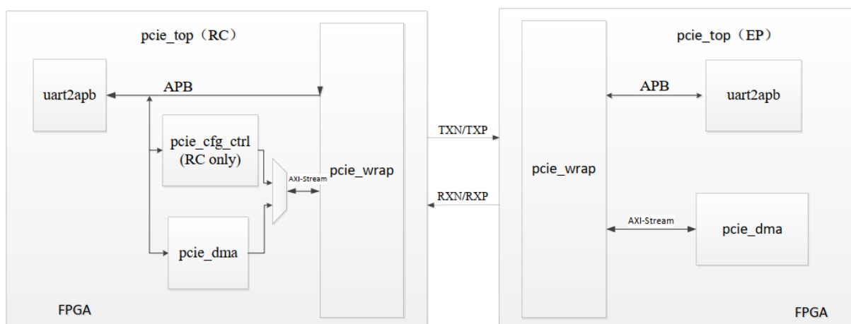
图 13 仿真参考设计功能框图
