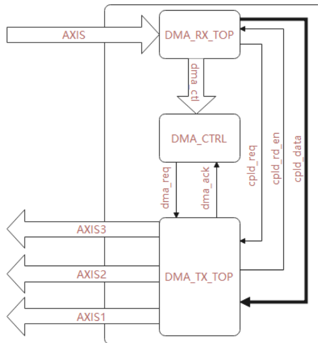
图 3 PCIe_DMA 模块内部框图
