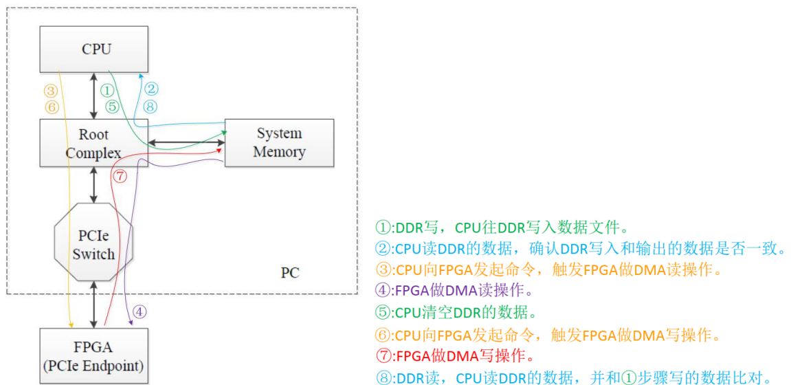
图 4 DMA 操作流程
