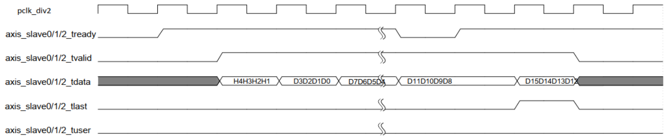
图 8 4DW Posted 操作时序
