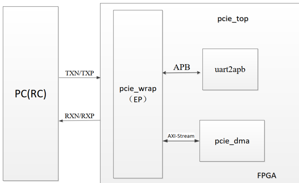
图 2 PCIe DMA 功能框架图
