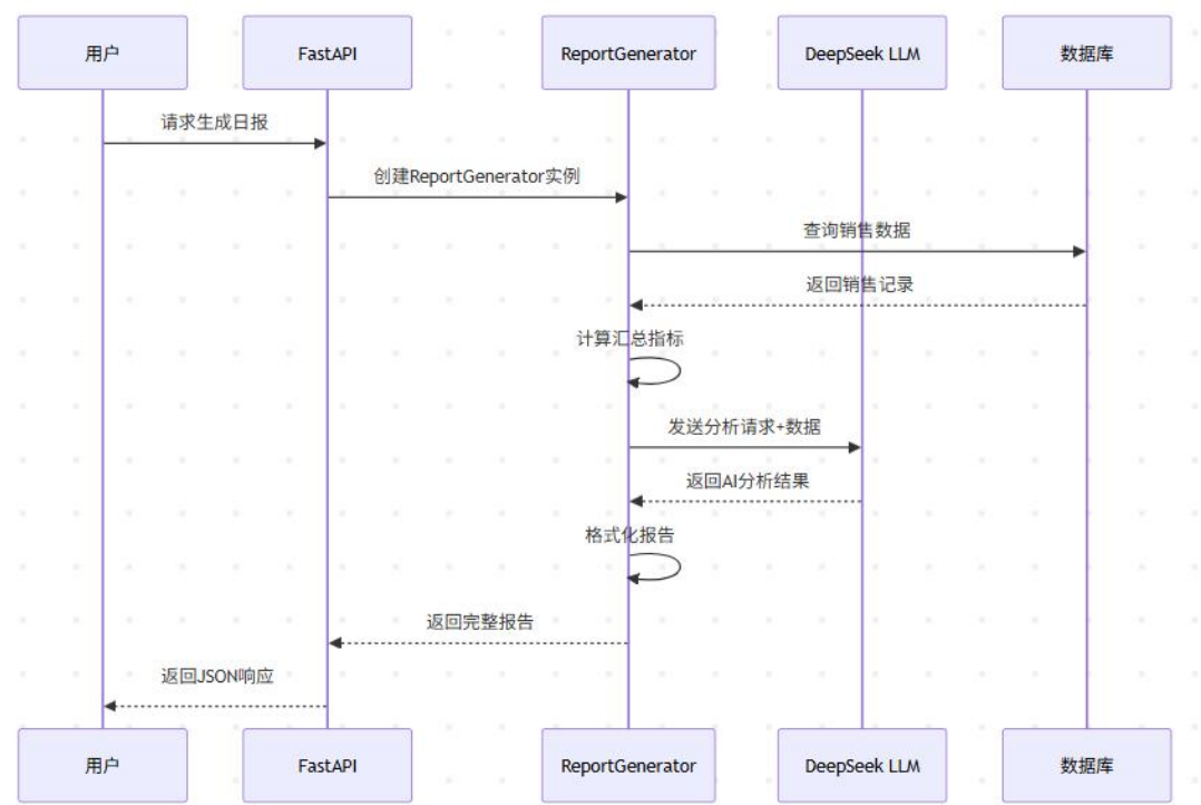
图 3.2 智能报表 Agent 工作流程
