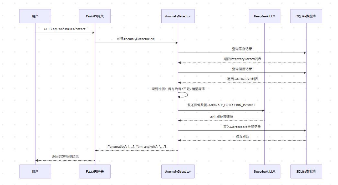
图 3.3 异常检测 Agent 工作流程
