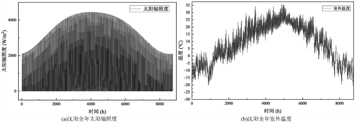
图 2.8 沈阳全年逐时气象参数
