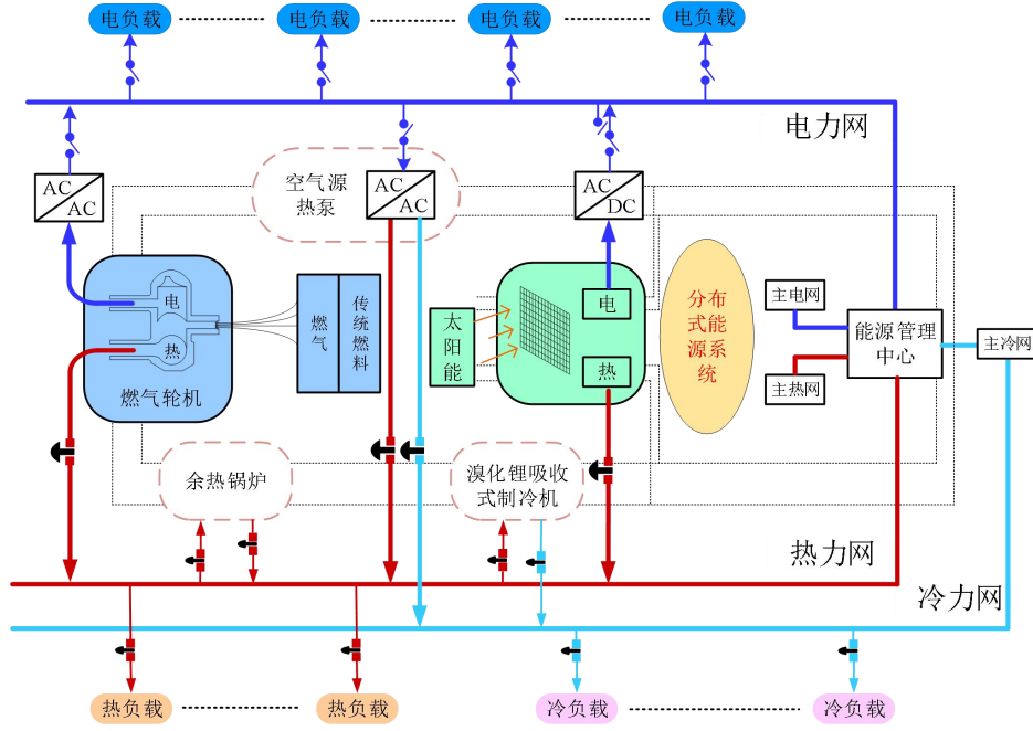
图 4.2 SH-CCHP 系统架构图
