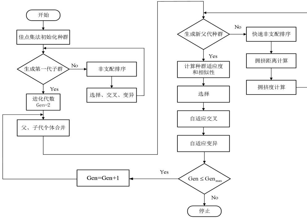
图 4.6 改进的 NSGA-II 算法 Figure 4.6 Improved NSGA-II algorithm
