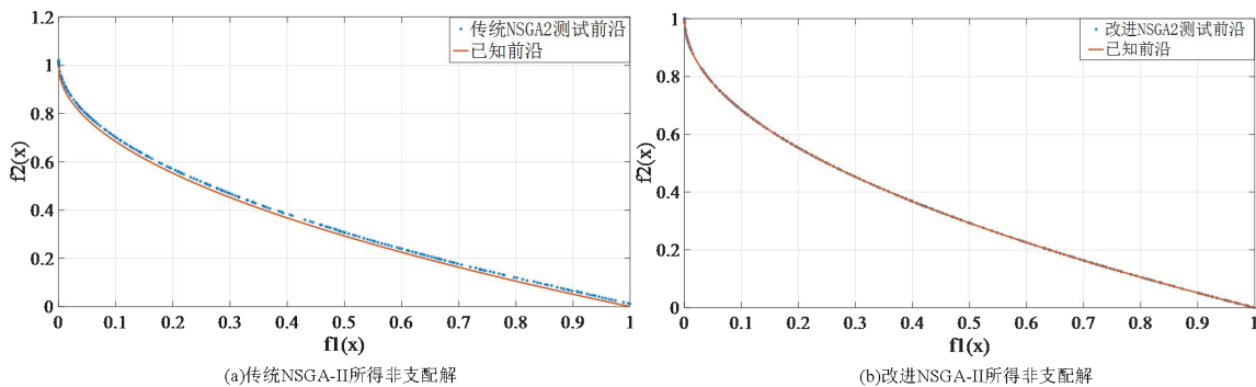
图 4.8 ZDT1 测试结果
