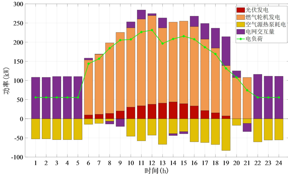
图 4.19 夏季典型日的供电运行策略
