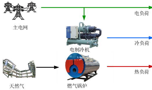
图 4.3 传统分离系统
