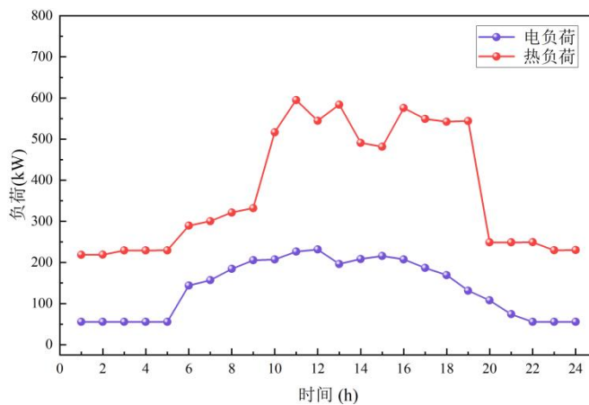
图 2.12 冬季典型日负荷
