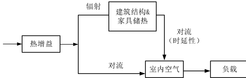
图 2.7 瞬时热增益与瞬时负载间的关系
