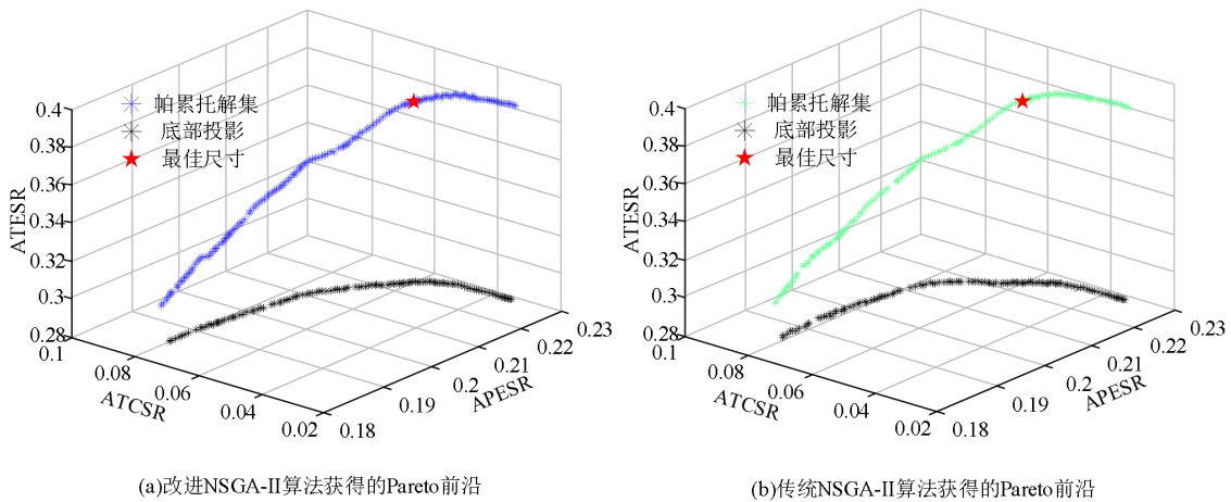
图 4.18 改进的 NSGA-II 算法获得的 Pareto 前沿
