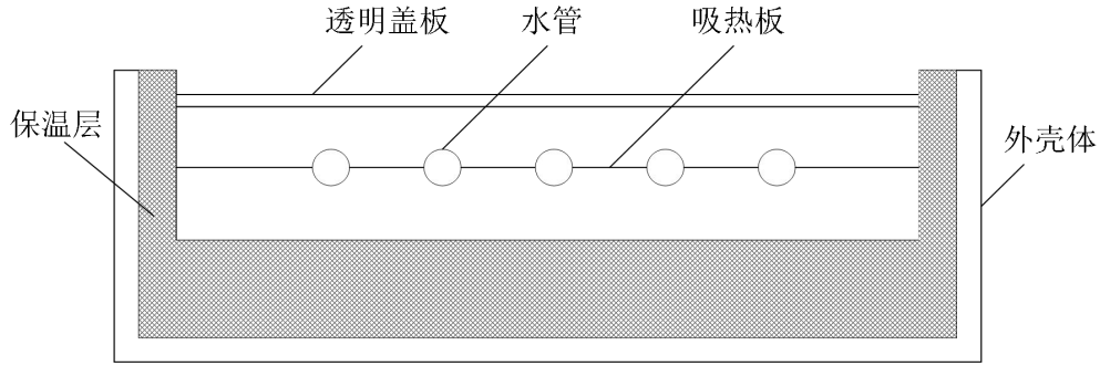
图 3.9 平板型太阳能集热器示意图
