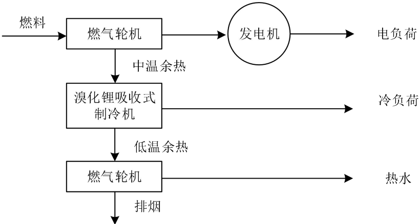
图 1.2 典型分布式冷热电联供系统
