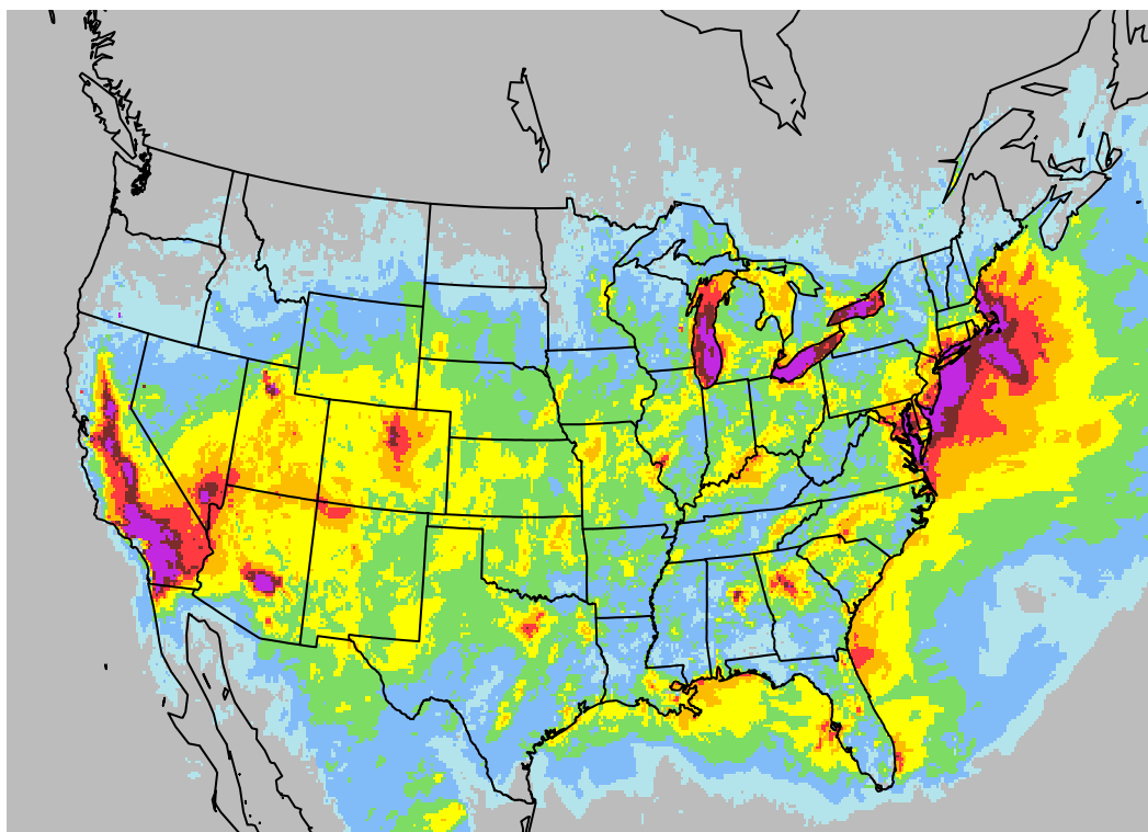
CMAQ
