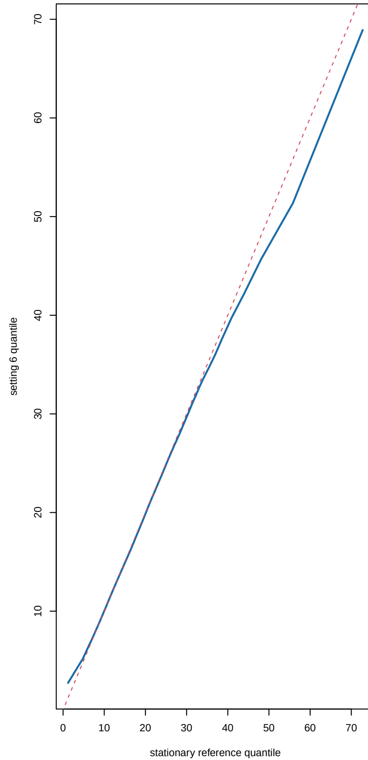
6 covdep_cov
