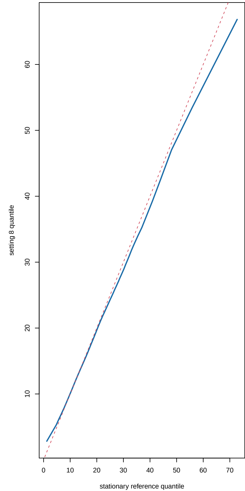
8 fuentes_cov
