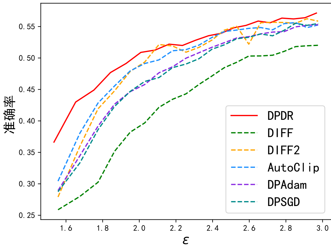
CIFAR10
