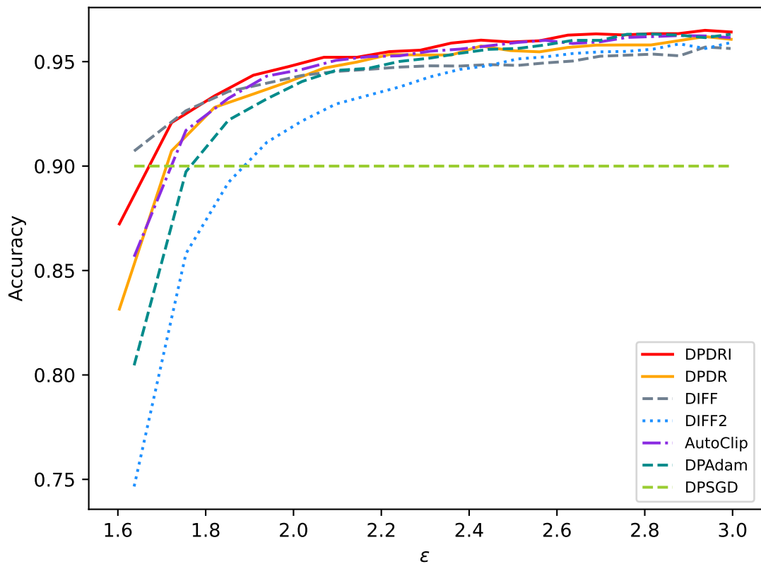
MNIST \varepsilon=3
