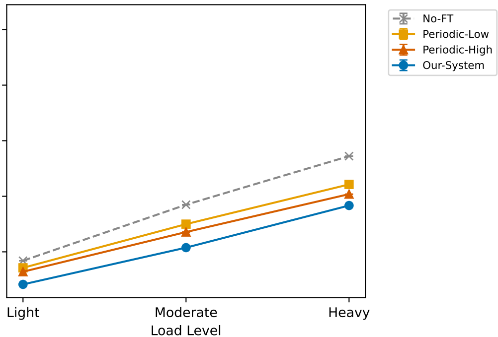
W4 Mixed
