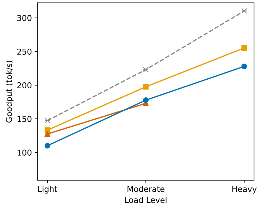
W1 Chat
