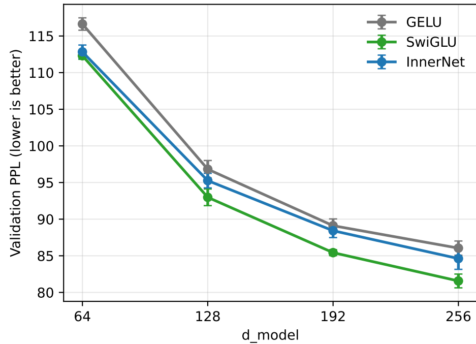
WikiText-2 Transformer FFN (same width)
