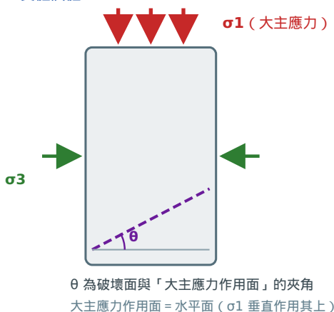
實體試體
