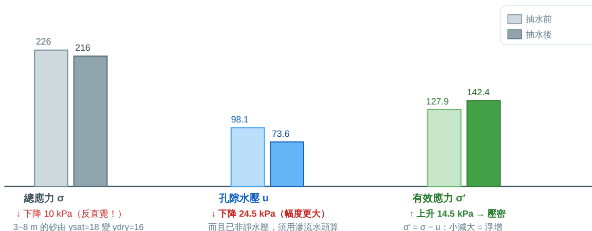
抽水前後（黏土層中央點，地表下 13 m）
