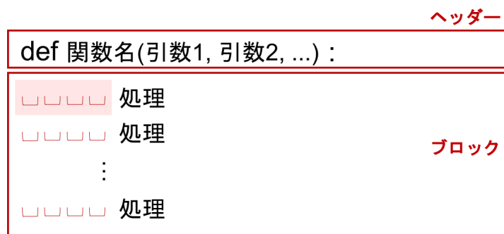
図 3.5 関数の定義
