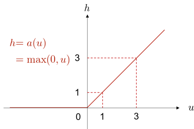
図 18.10 ReLU 関数
