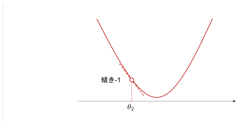
図 5.2 微分 2
