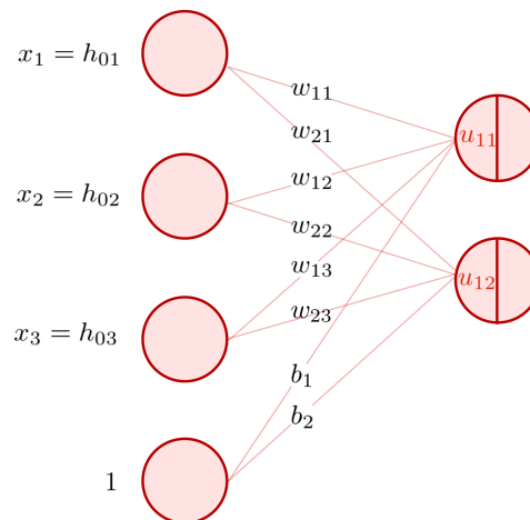
図 18.5 線形変換
