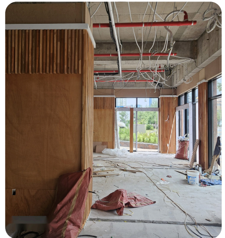
합판 바탕 위 각재 고정
