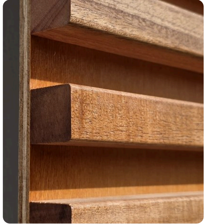
합판 바탕 단면 — 합판 위 30×30 각재, 30mm 간격 접착·고정 · 바탕 합판은 원하는 색상으로 도장 가능
