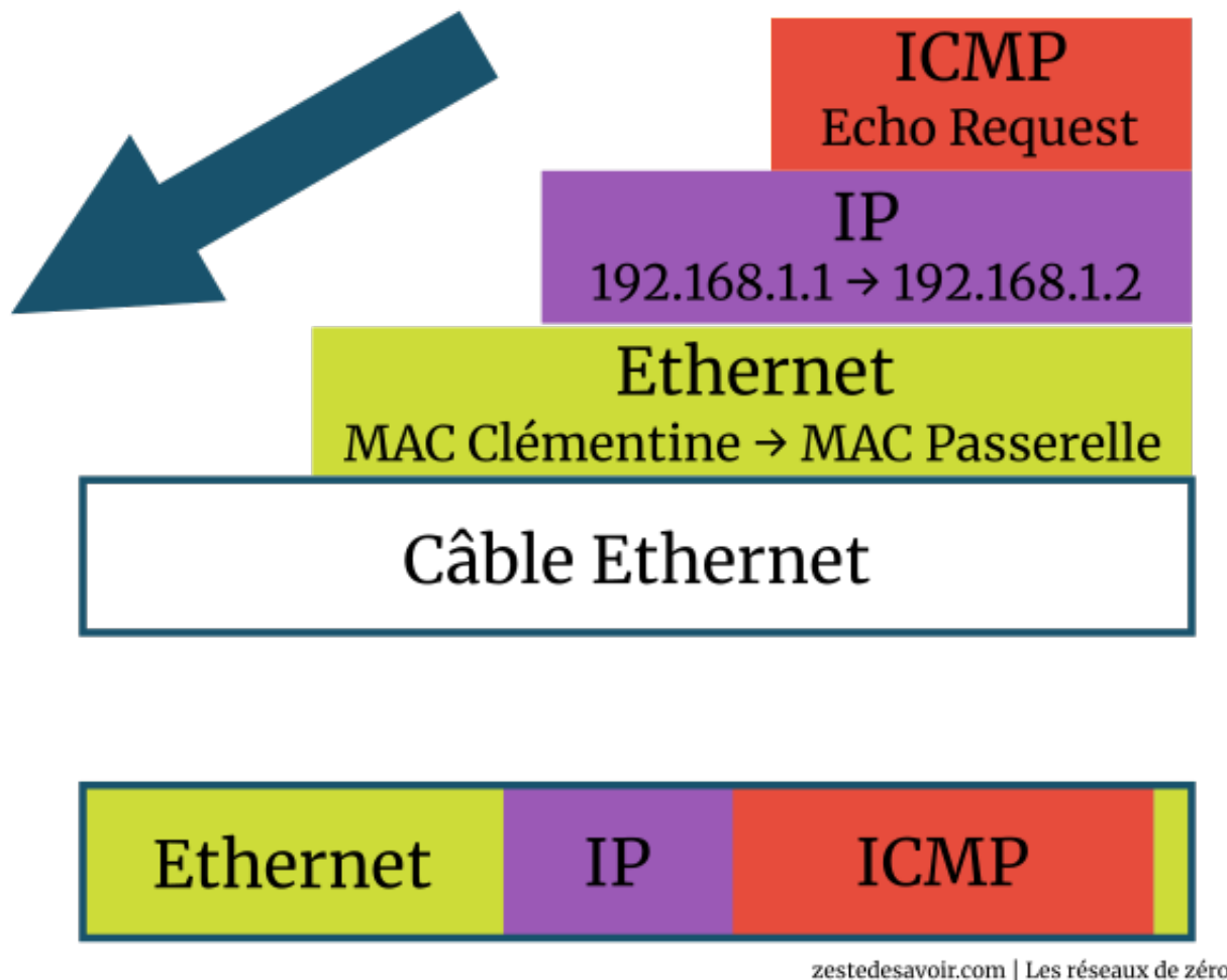
FIGURE V.3.1. – Un paquet simplement encapsulé dans Ethernet (CC BY)
