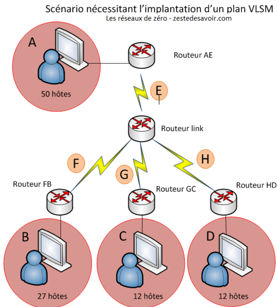
FIGURE III.6.1. – Scénario nécessitant l'implantation d'un plan VLSM
