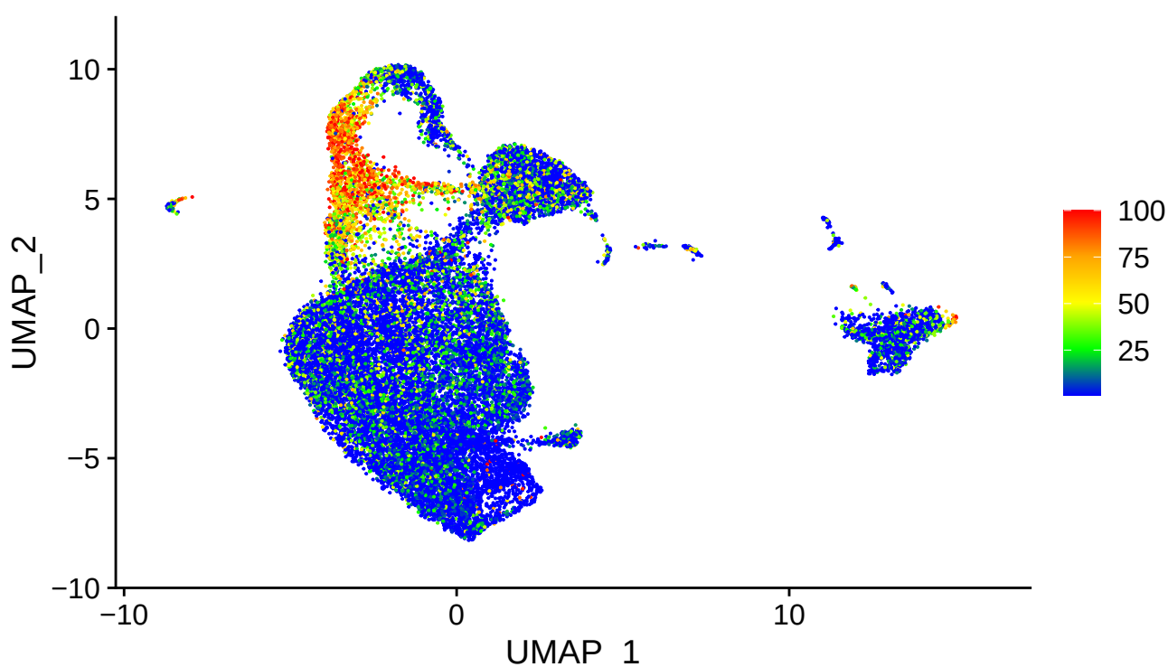
KRT14
