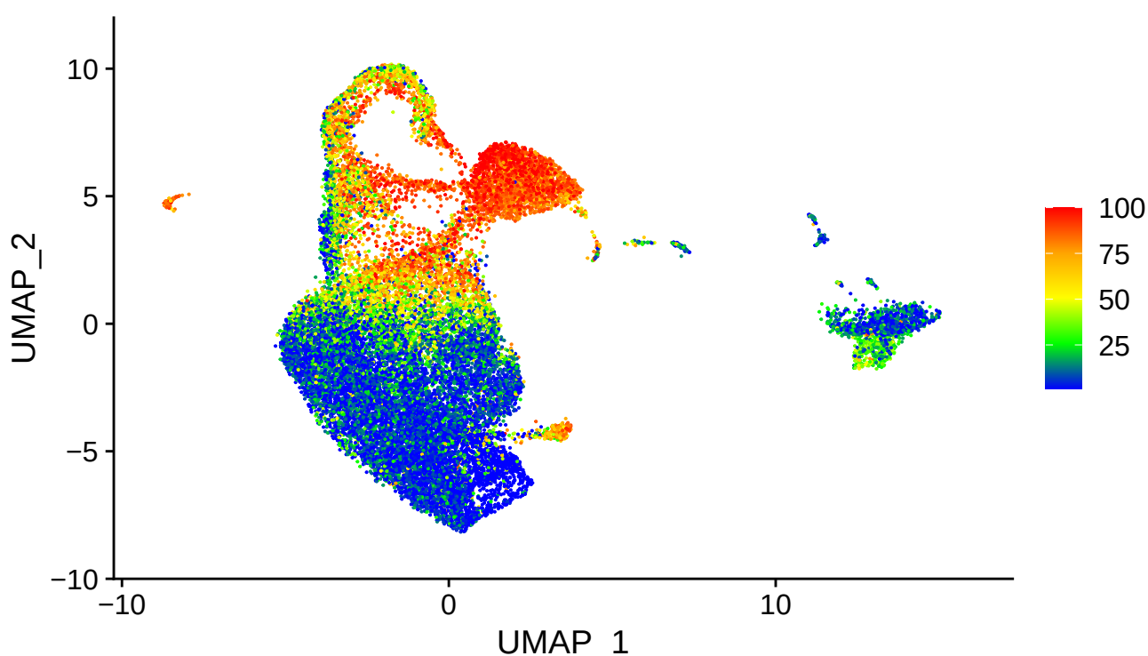
KRT5
