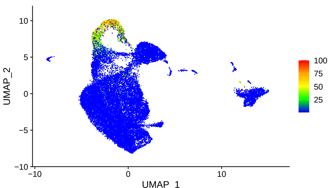
CCNB1
