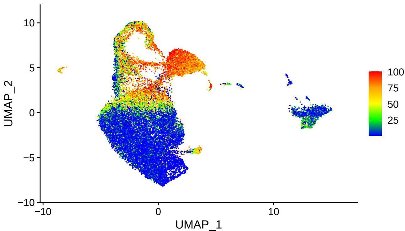
KRT15
