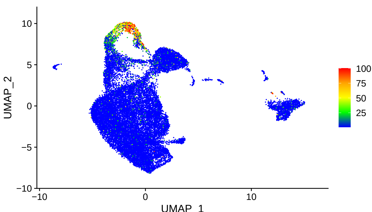
PCNA
