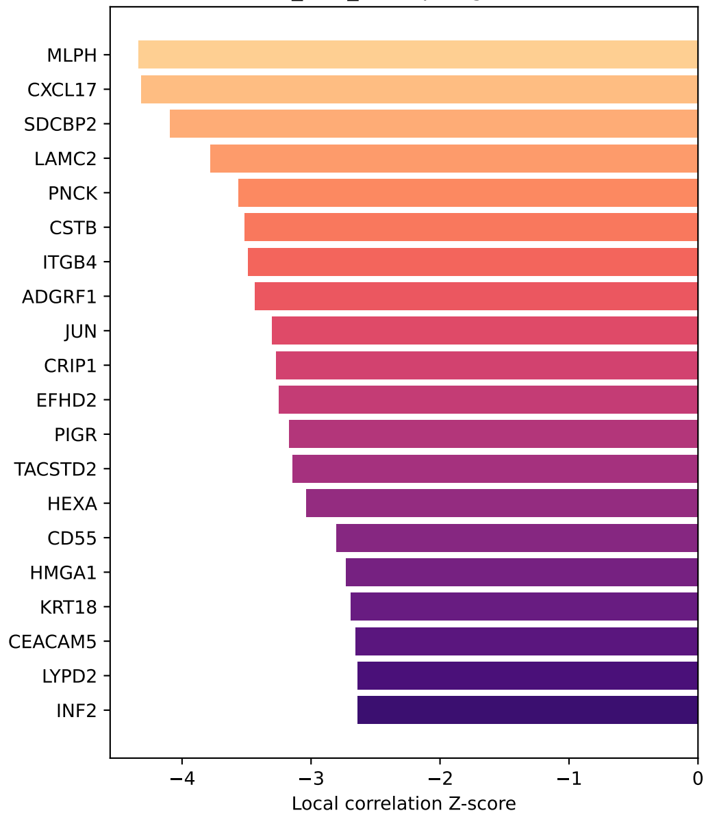
IU_PDA_T8: top negative
