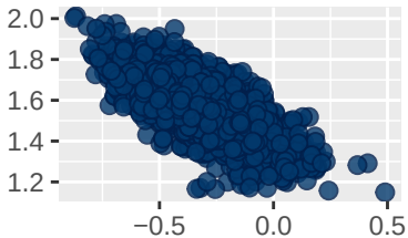
b_drug1
