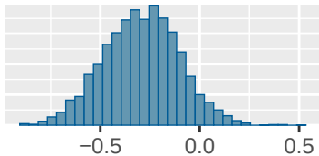
b_drug1
