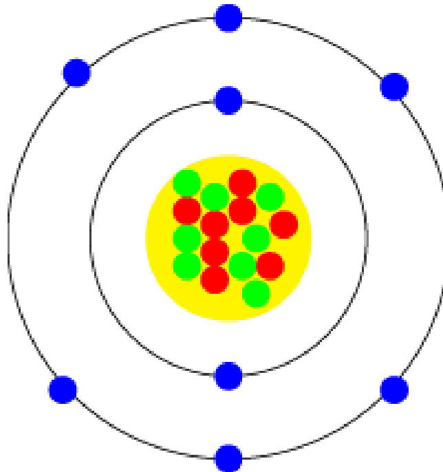
Modelo atômico de Bohr — níveis de energia do elétron
