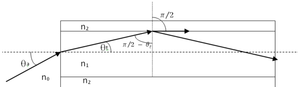
Ângulo de aceitação em fibras ópticas — óptica geométrica
