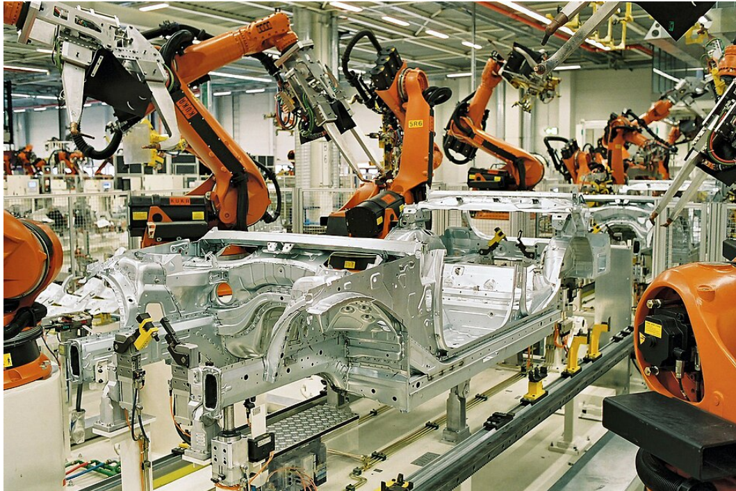
BMW Leipzig MEDIA 050719 Download Karosseriebau max
