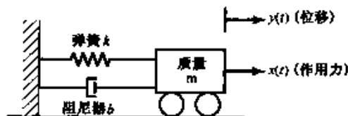
图 6.21 由弹簧、减振器及一个连接着它们的可移动质量和一个固定支撑组成的二阶系统
