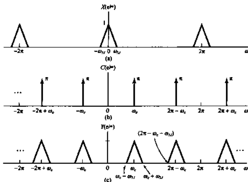
图 8.42 利用正弦载波的高散时间幅度调制的有关频谱。(a) 带限信号 x[n] 的频谱; (b) 正弦载波信号 c[n] = \cos \omega_c n 的频谱; (c) 已调信号 y[n] = x[n]c[n] 的频谱
