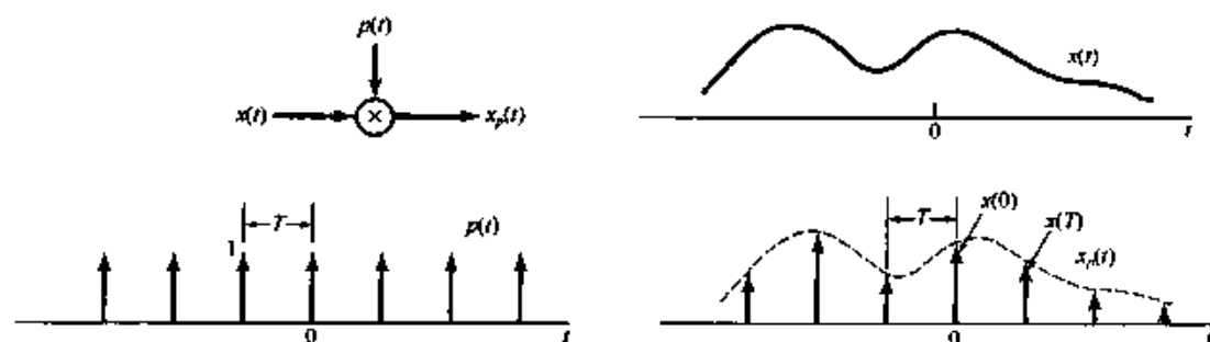
图 7.2 冲激串采样
