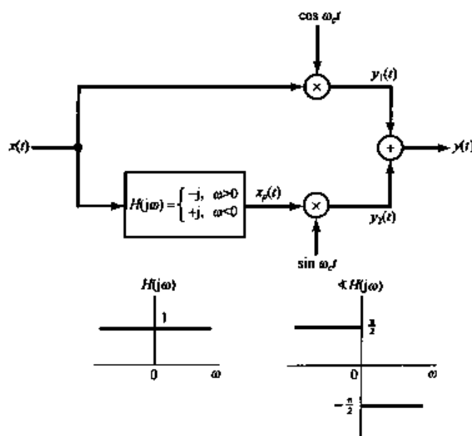
图 8.21 利用一个 90^\circ 相移网络, 仅保留下边带的单边带幅度调制系统
