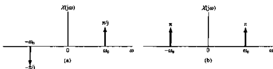
图 4.13 (a) x(t) = \sin \omega_0 t 的傅里叶变换; (b) x(t) = \cos \omega_0 t 的傅里叶变换
