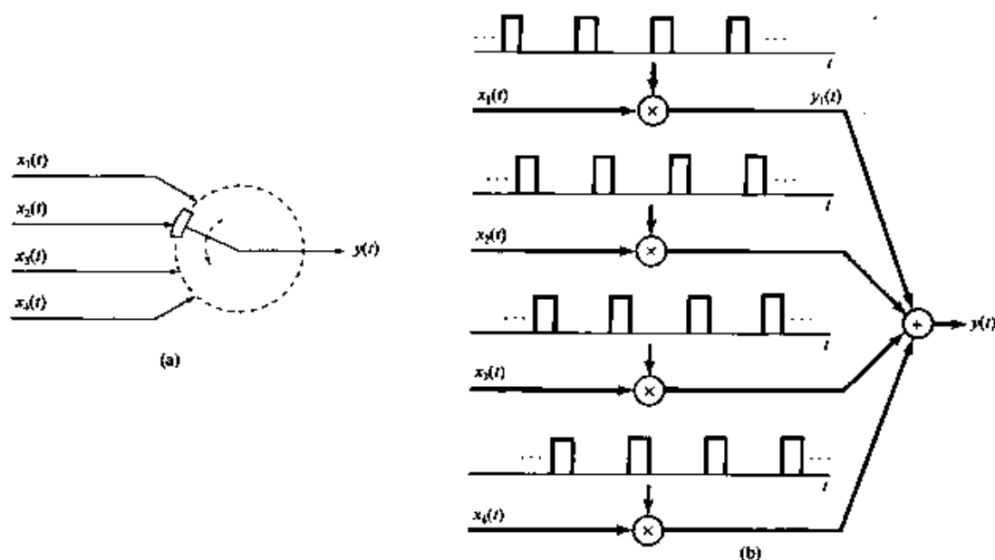
图 8.25 时分多路复用
