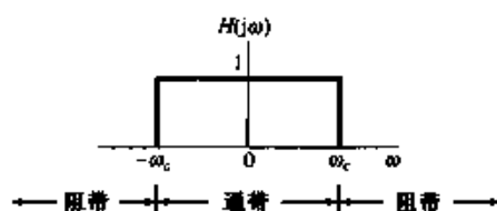
图 4.20 理想低通滤波器的频率响应
