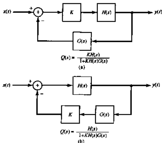
图 11.10 包含一个可调增益的反馈系统。(a) 可调增益位于正向通路的系统;(b) 可调增益位于反馈通路的系统
