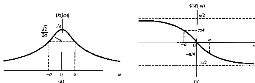
图 4.5 例 4.1 中信号 x(t) = e^{-\alpha}u(t) , \alpha > 0 的傅里叶变换
