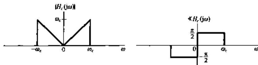
图 7.27 连续时间理想带限微分器的频率响应 H_c(j\omega) = j\omega, |\omega| < \omega_c
