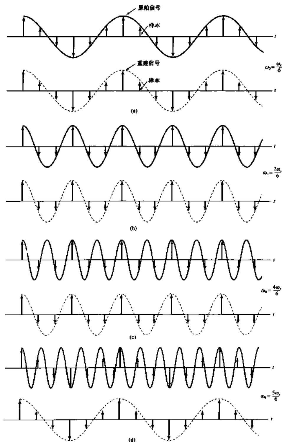
图 7.16 在一个正弦信号上混叠的效果。对应于 4 种不同的 \omega_0 值,画出了原始正弦信号 (实线),它的样本和重建信号 (虚线)。(a) \omega_0 = \omega_c/6 ; (b) \omega_0 = 2\omega_c/6 ; (c) \omega_0 = 4\omega_c/6 ; (d) \omega_0 = 5\omega_c/6 。在 (a) 和 (b) 中没有混叠发生,而在 (c) 和 (d) 中则存在混叠
