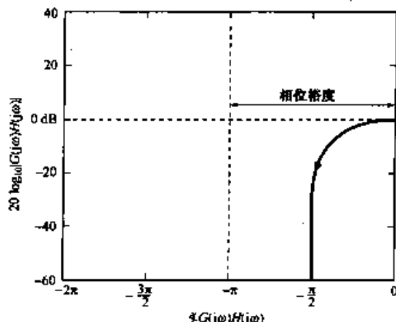
图 11.29 例 11.10 所示一阶系统的对数幅-相图
