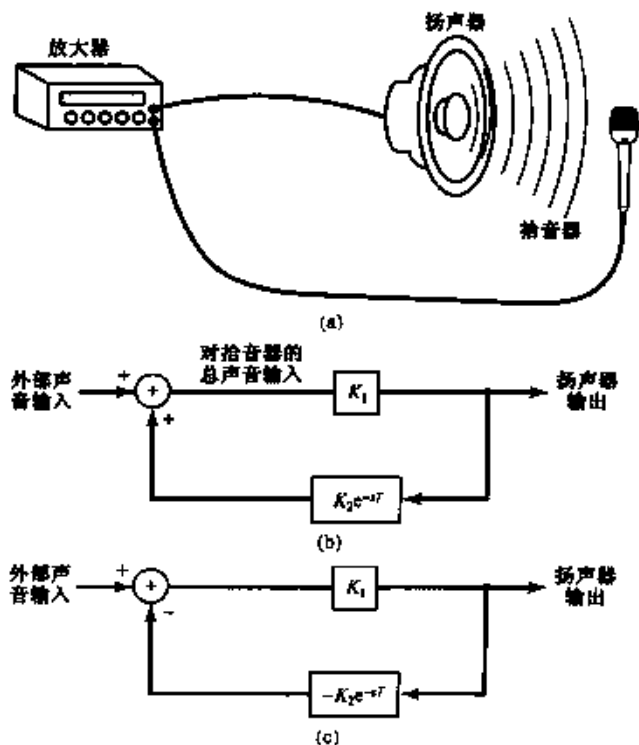
图 11.8 (a) 音频反馈现象的形象表示; (b) 图(a)的方框图表示; (c) 将(b)的方框图画成一个负反馈系统(注意: e^{-sT} 就是 T 秒延迟环节的系统函数)
