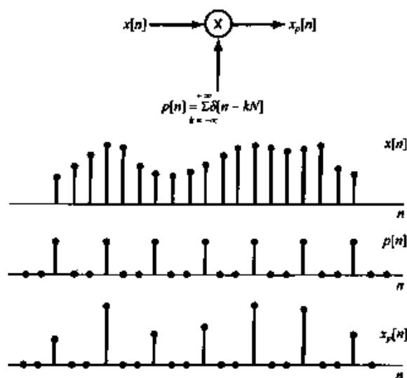
图 7.31 离散时间采样
