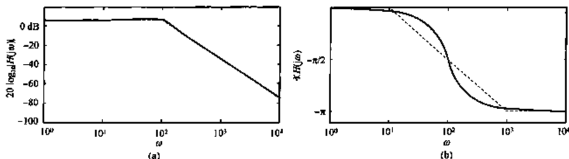
图 6.24 例 6.4 的系统函数伯德图。(a) 模; (b) 相位
