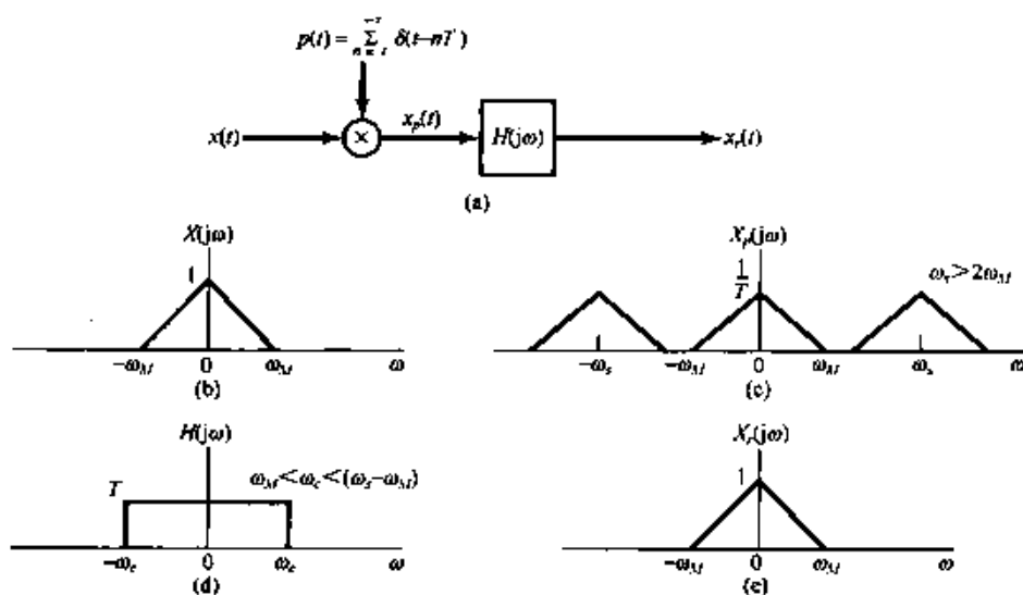
图7.4 利用一个理想低通滤波器从信号的样本中完全恢复一个连续时间信号。(a) 采样与恢复系统;(b) x(t) 的频谱;(c) x_p(t) 的频谱;(d) 用于从 X_s(j\omega) 恢复 X(j\omega) 的理想低通滤波器;(e) x_r(t) 的频谱
