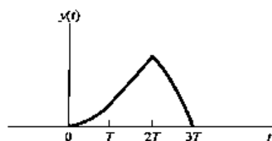
图 2.21 例 2.7 中信号 y(t) = x(t) * h(t)
