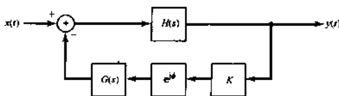
图 11.26 在图 11.25 的标称系统中，包括可能的增益和相位偏移的反馈系统
