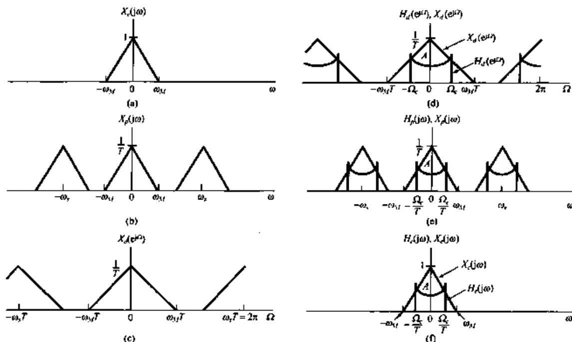
图 7.25 图 7.24 所示系统的频域说明。(a) 连续时间信号的频谱 X_c(j\omega) ;(b) 冲激串采样以后的谱; (c) 离散时间序列 x_d[n] 的谱;(d) H_d(e^{j\Omega}) 和 X_d(e^{j\Omega}) 相乘后得到的 Y_d(e^{j\Omega}) ;(e) H_p(j\omega) 和 X_p(j\omega) 相乘后得到的 Y_p(j\omega) ;(f) H_c(j\omega) 和 X_c(j\omega) 相乘后得到的 Y_c(j\omega)
