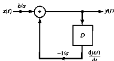
图 2.30 利用相加器、乘以系数和微分器的式(2.128)和式(2.129)所示系统的方框图表示
