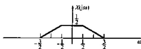
图 4.25 例 4.23 中 x(t) 的傅里叶变换
