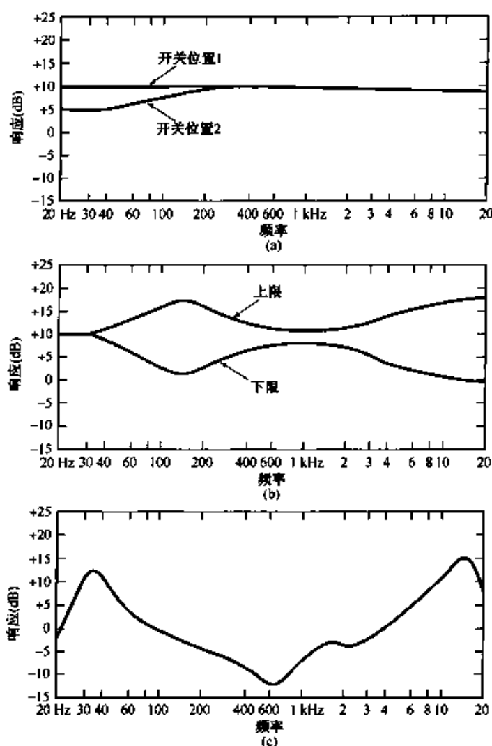
图 3.22 用于一组特殊音频扬声器系统中的均衡器电路频率响应的模型特性,图中示出为 20 \log_{10} |H(j\omega)| , 单位 dB。(a) 用双位开关控制的低频滤波器;(b) 连续可调成形滤波器频率响应的上、下限特性范围;(c) 均衡器级的固定频率响应
