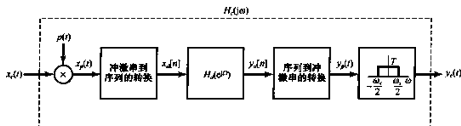
图 7.24 利用离散时间滤波器过滤连续时间信号的系統
