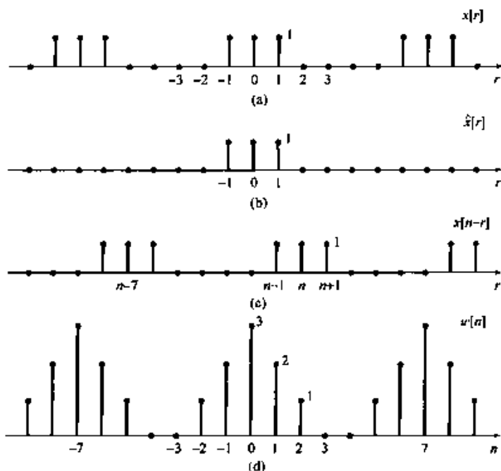
图 3.21 (a) 例 3.15 中的方波序列 x[r] ; (b) 序列 \tilde{x}[r] , -3 \leq r \leq 3 时 \tilde{x}[r] = x[r] , 对于其余 r , \tilde{x}[r] = 0 ; (c) 序列 x[n-r] ; (d) 序列 w[n] 等于 x[n] 与其本身的周期卷积, 也等于 \tilde{x}[n] 与 x[n] 的非周期卷积
