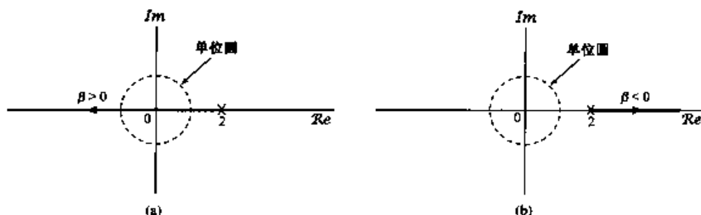
图 11.9 随 \beta 值变化,由式(11.40)表示的闭环系统的极轨迹。(a) \beta > 0 ; (b) \beta < 0 。注意:图中已标出 z=2 的点,它对应于 \beta=0 的极点位置
