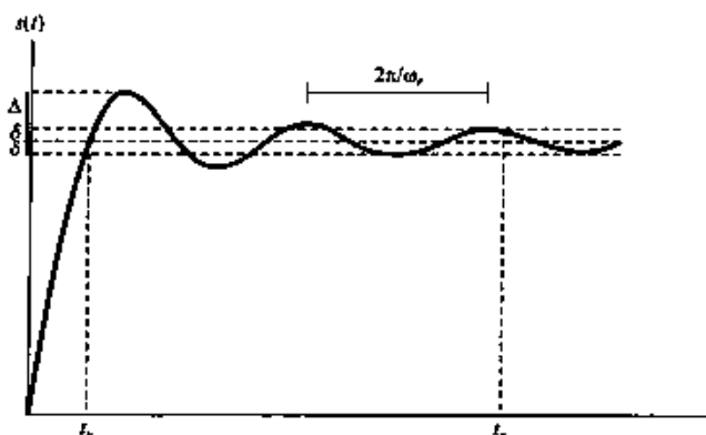
图 6.17 一个连续时间低通滤波器的阶跃响应,图中指出上升时间 t_r , 超量 \Delta , 振荡频率 \omega , 和建立时间 t_s , 即阶跃响应位于其终值 \pm \delta 内所需要的时间
