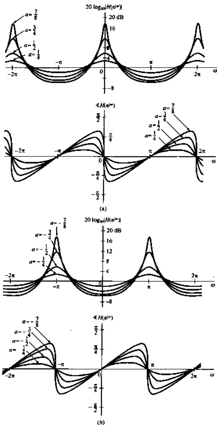
图 6.28 由式(6.52)确定的一阶系统频率响应的模和相位特性。
