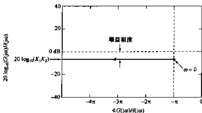
图 11.32 例 11.12 的对数幅-相图
