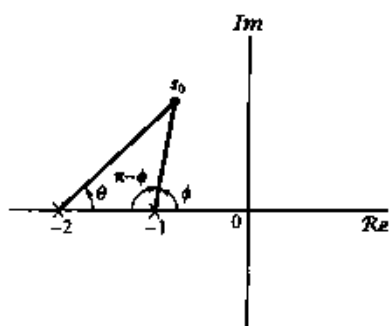
图 11.11 例 11.1 中求满足角判据的几何方法
