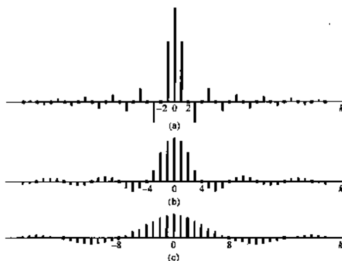
图 3.7 在某一固定的 T_1 值和几个不同的 T 值时, 周期性方波傅里叶级数系数 Ta_k 的图。(a) T=4T_1 ; (b) T=8T_1 ; (c) T=16T_1 。这些系数都是包络 (2\sin\omega T_1)/\omega 的等间隔样本, 样本间隔为 2\pi/T , 随 T 的增加而减小
