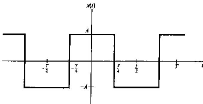
图 8.36 对称周期方波
