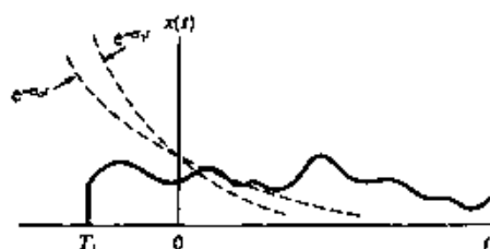
图 9.7 若 x(t) 是右边信号, 而 x(t)e^{-\sigma_1 t} 是绝对可积的, 那么 x(t)e^{-\sigma_1 t} , \sigma_1 > \sigma_0 也一定绝对可积
