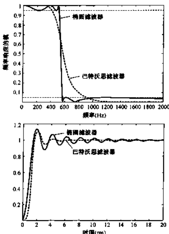
图 6.18 具有相同通带和阻带波纹, 相同截止频率的五阶巴特沃思滤波器和五阶椭圆滤波器的例子。(a) 频率响应的模特性; (b) 阶跃响应
