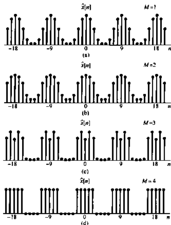
图 3.18 图 3.16 中的周期方波序列的部分和表示, 即式(3.106)和式(3.107), 在 N=9 和 2N_1+1=5 时对应于几个不同 M 值时的波形。(a) M=1 ; (b) M=2 ; (c) M=3 ; (d) M=4
