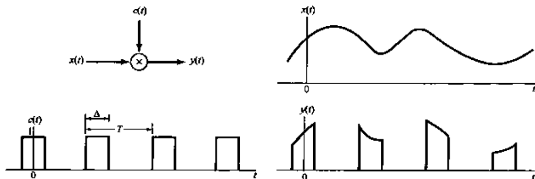
图 8.23 脉冲串幅度调制
