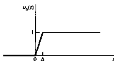
图1.33 单位阶跃的连续近似 u_{\Delta}(t)
