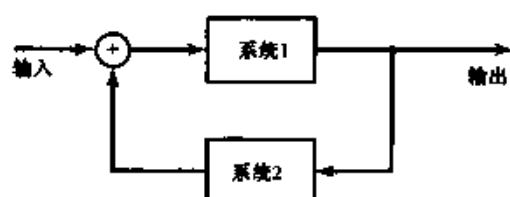
图 1.43 反馈互联
