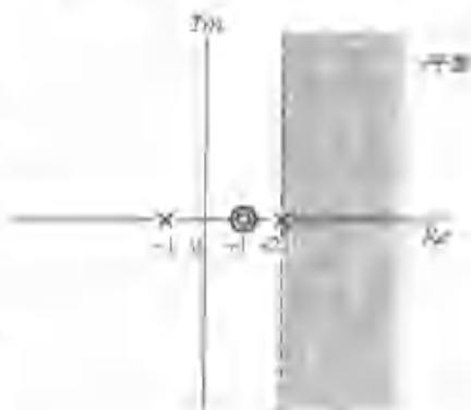
图 9.3 例 9.5 的零-极点图和收敛域
