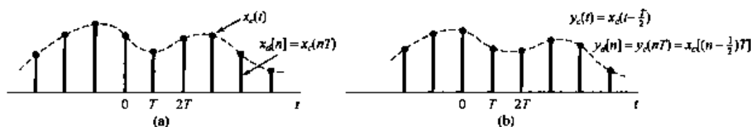
图 7.30 (a) 连续时间信号 x_c(t) 的样本序列; (b) 在 (a) 中延时半个采样间隔的序列
