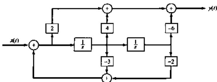
图 9.35 例 9.31 系统的直接型表示
