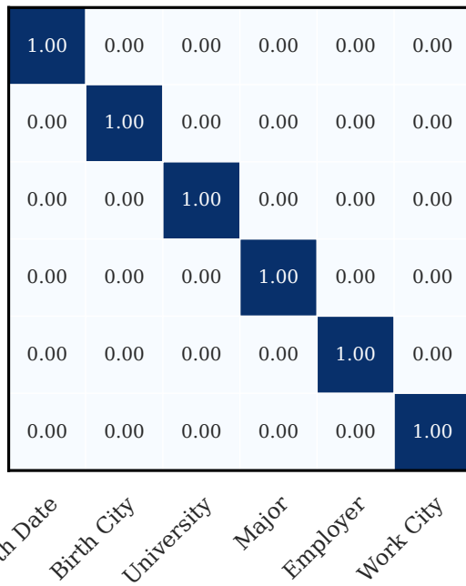
(b) Layer 6
