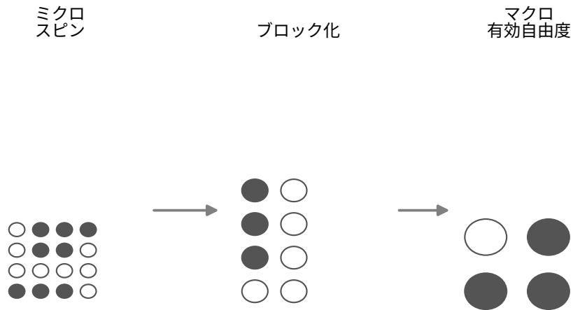
(a) 物理：粗視化 (RG)
