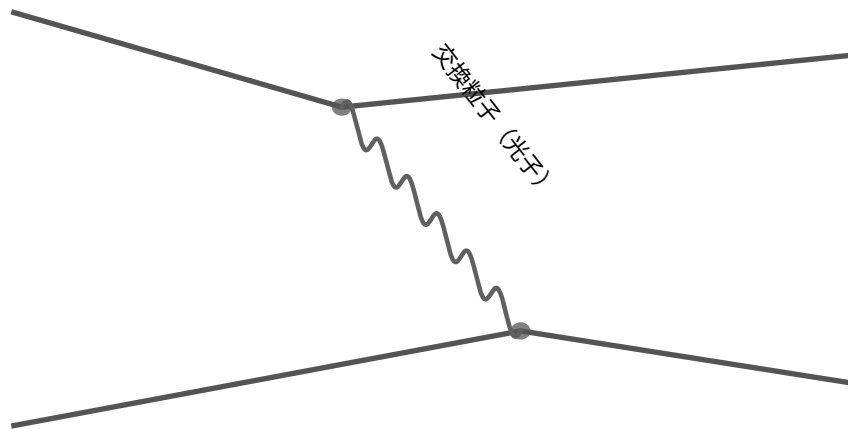
(a) 物理：ファインマン・ダイアグラム
