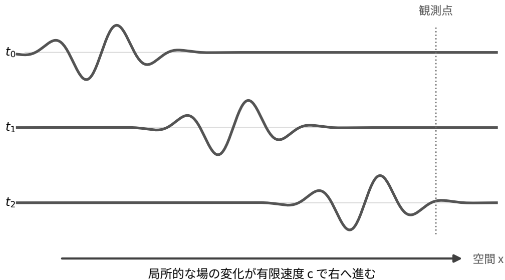
(a) 物理：電磁波は空間を伝播する
