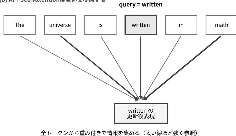
(b) AI：Self-Attentionは全体を参照する
