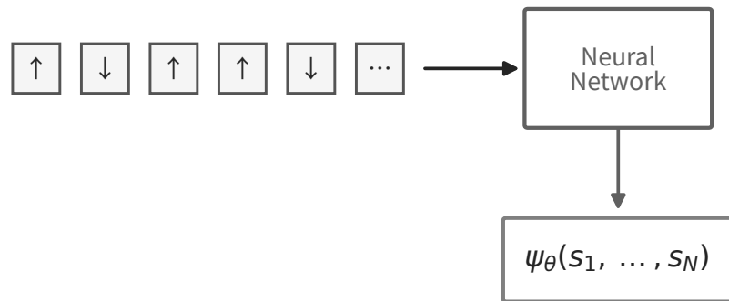
(b) NNQS : 巨大な波動関数を関数として圧縮
