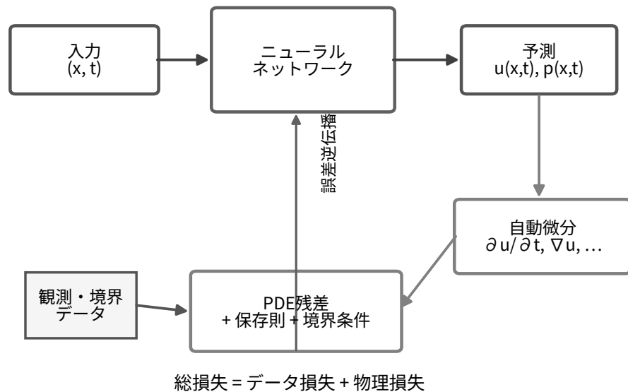
(a) PINN の学習ループ
